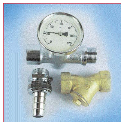
T-Stück mit Thermometer Direktanschluss für Schläuche und Schmutzfänger
