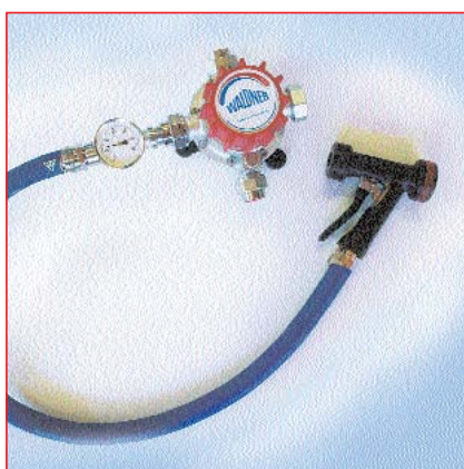
Typ 2000 mit T-Stück und Thermometer sowie Schlauch und Pistole
