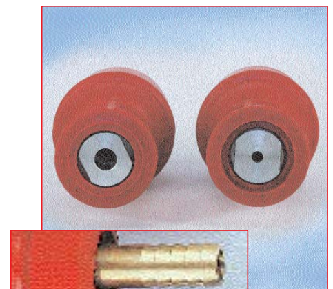
links 10 mm Austrittsdüse rechts 5 mm Austrittsdüse 3/4"-Schlauchstutzen standard
