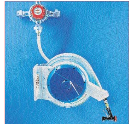
Schlauchaufroller mit Aluminium- oder Kunststoffgehäuse
